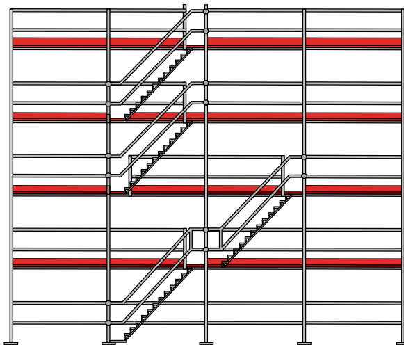
5 Escaliers d'échafaudage corrects: la volée continue est limitée à deux longueurs de ponts d'échafaudage.
