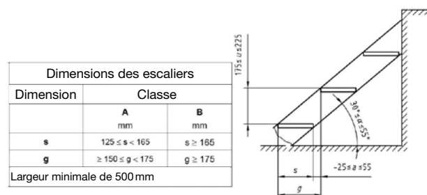
2 Dimensions d'escaliers selon le point 5.8 SN EN 12811-1: 2003
