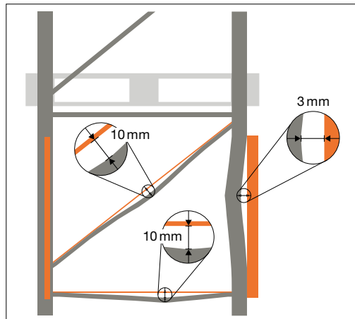
2 Maximal zulässige Beschädigungen an Regalstützen und Verstrebungen; Grenzwerte gemäss SN EN 15635.
