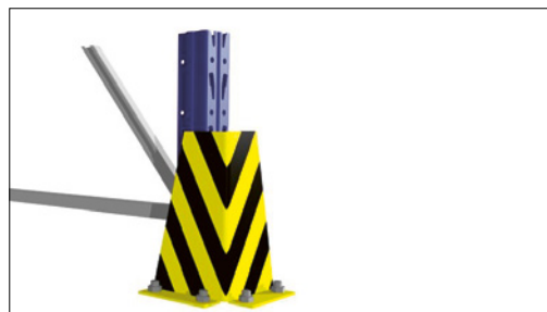
1 Anfahrsschutz an den Ecken der Regale (Mindesthöhe 30 cm, empfohlen 40 cm oder grösser; am Boden festgeschraubt und nicht mit dem Regal verbunden).
