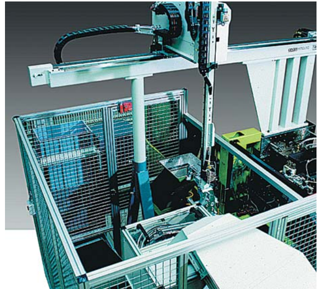
Manipolatore industriale
