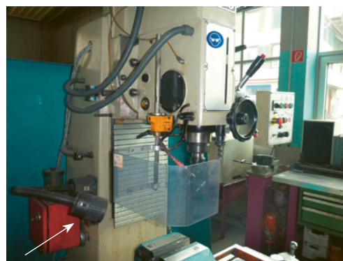
2 Una lampada locale (a sinistra) permette di ottenere un'illuminazione ottimale intorno al trapano.
