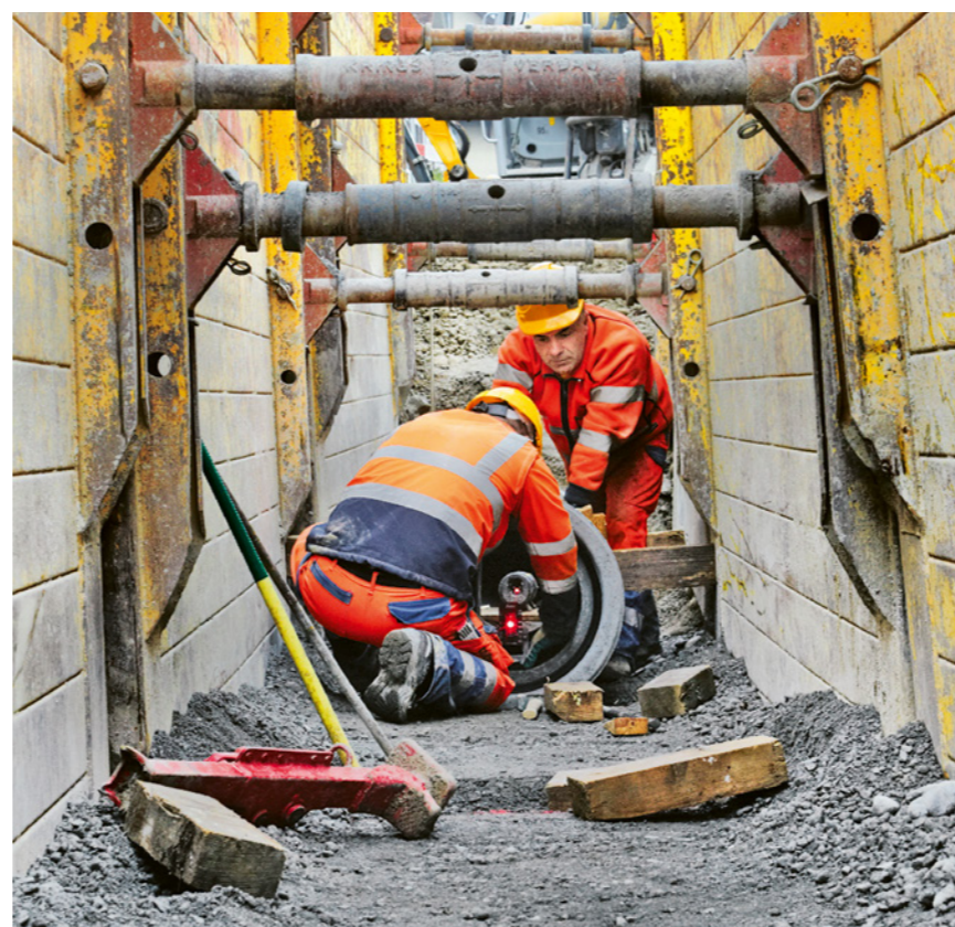
Regola 8: mettiamo in sicurezza gli scavi a partire da una profondità di 1,5m.
