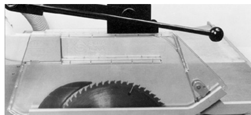
1 Cuffia di protezione a scorrimento parallelo con copertura per lama incisore
