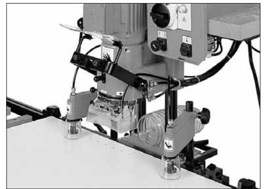
Foto 3: cilindri pneumatici schermati da una cuffia di protezione.
