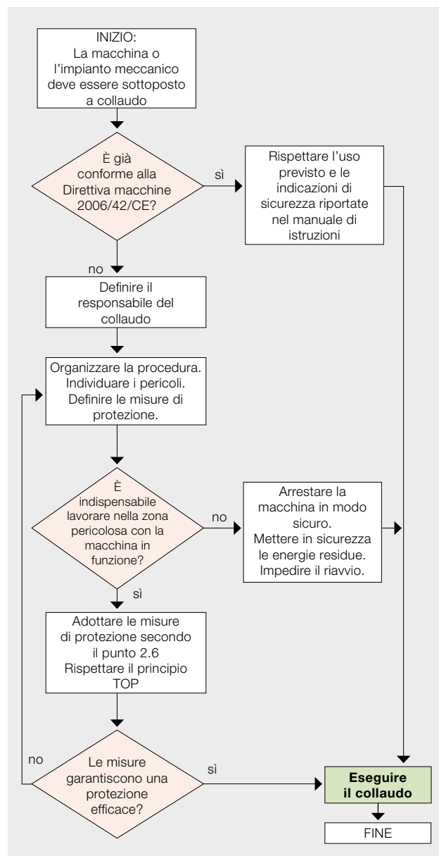
Fig. 2: diagramma di flusso del collaudo
