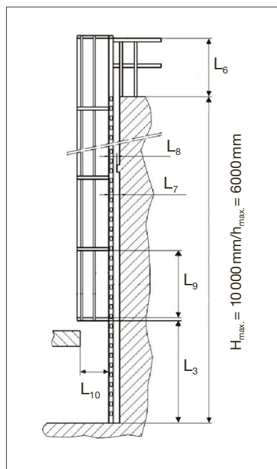
4 Vue latérale d'une échelle fixe (schéma: SN EN ISO 14122-4)
