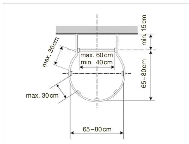
3 Échelle à crinoline vue d'en haut
