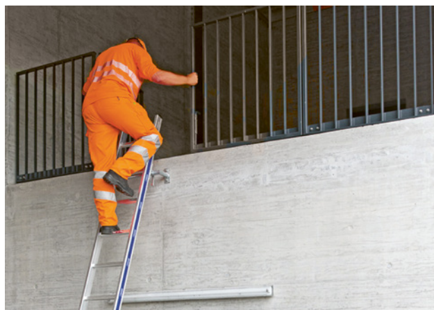
33 Dispositivo per tenersi, parapetto in prossimità dell'apertura nel vuoto ed estremità superiore della scala messa in sicurezza
