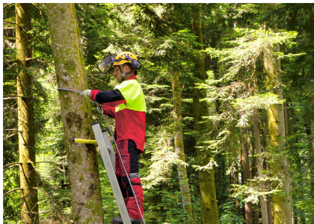
46 Scala con staffa antiribaltamento
