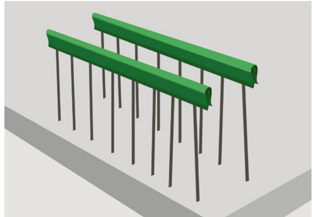
3 Abdeckung der Anschlussbewehrung mit geprüfem Schutzprofil
