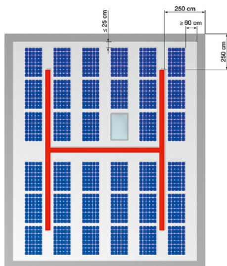
9 Esempio di forma ad H
