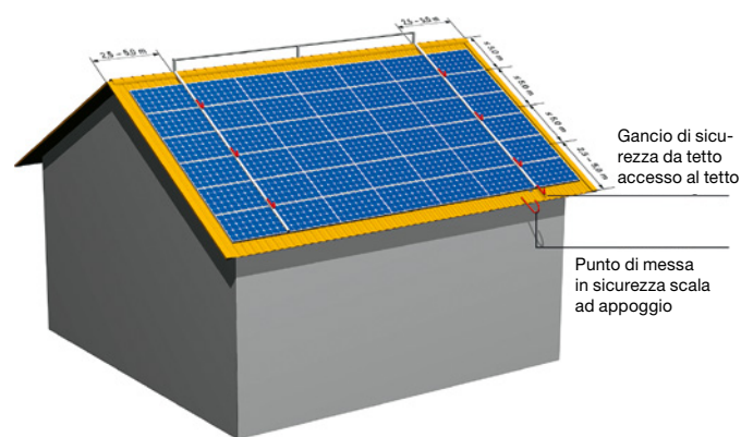
18 Esempio di protezione dalle cadute con sistema per dispositivi anticaduta sul colmo, combinata con ganci di sicurezza da tetto.
