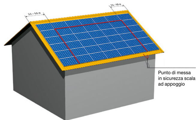
19 Esempio di protezione anticaduta con sistema a binari. Nota: il sistema a binario deve essere previsto dal fabbricante in base all'inclinazione del tetto.
