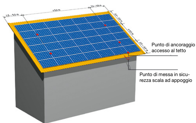
16 Esempio di protezione anticaduta con ancoraggi a punto singolo per pannelli solari calpestabili (ad es. su un tetto a una falda).
