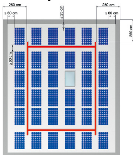
8 Esempio di forma a omega
