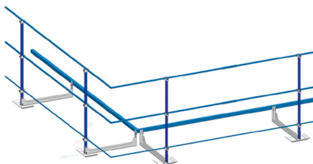
6 Parapetto senza perforazione del manto di copertura, stabilizzato alla struttura portante dell'impianto fotovoltaico
