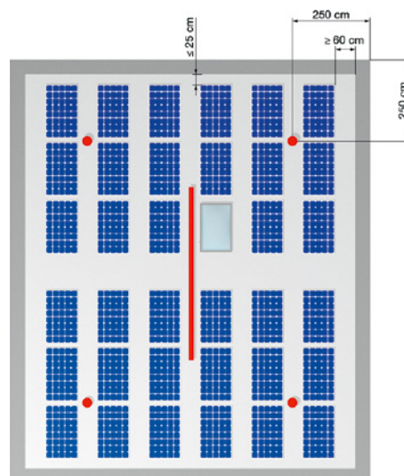
10 Esempio di forma a I, quando non è possibile realizzare la forma a omega o ad H.
