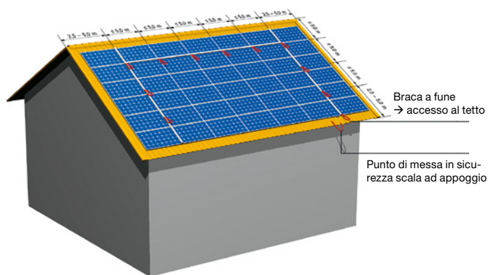
17 Esempio di protezione anticaduta con brache a fune di acciaio inossidabile (attenzione: evitare l'ombreggiamento), adatto per tetti con inclinazione fino a 40°.
