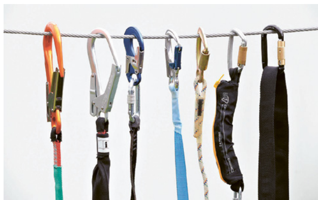
12 Moschettoni di sicurezza di vario tipo
