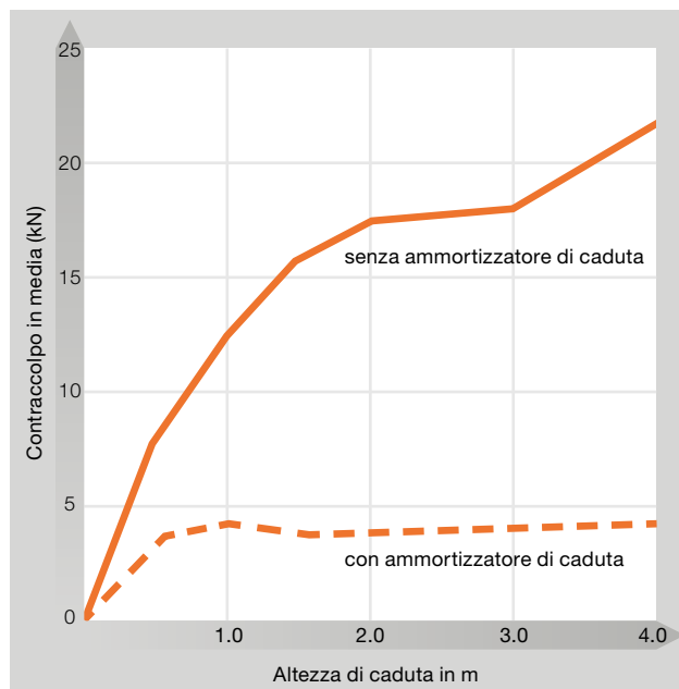
2 Contraccolpo in funzione dell'altezza di caduta durante le prove eseguite
