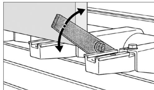
3 La pièce est maintenue au moyen d'un taquet.
