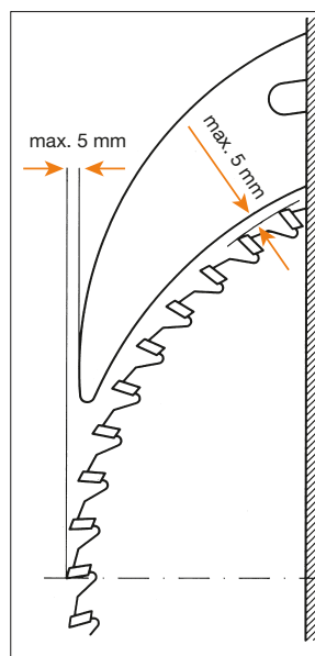
2 Couteau diviseur en position de sécurité correctement réglé.
