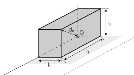
Fig. 5 Exemple pour un parallélépipède de référence sur trois plans réfléchissants et distance caractéristique d_0 par rapport au centre du système de coordonnées.
