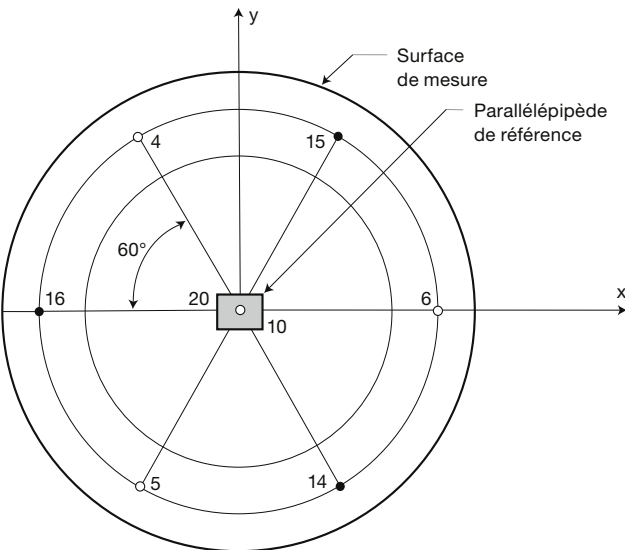
Fig. 6 Positions des microphones principaux 4, 5, 6 et 10 sur une surface de mesure hémisphérique (coordonnées: voir tableau 6).
