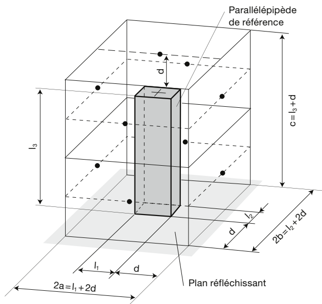
Fig. 10 Exemple de surface de mesure et de positions des microphones pour une machine haute à petite surface de base.
