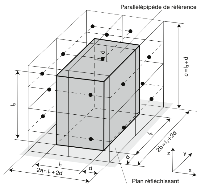
Fig. 12 Exemple de surface de mesure et de positions des microphones pour une machine moyenne.
