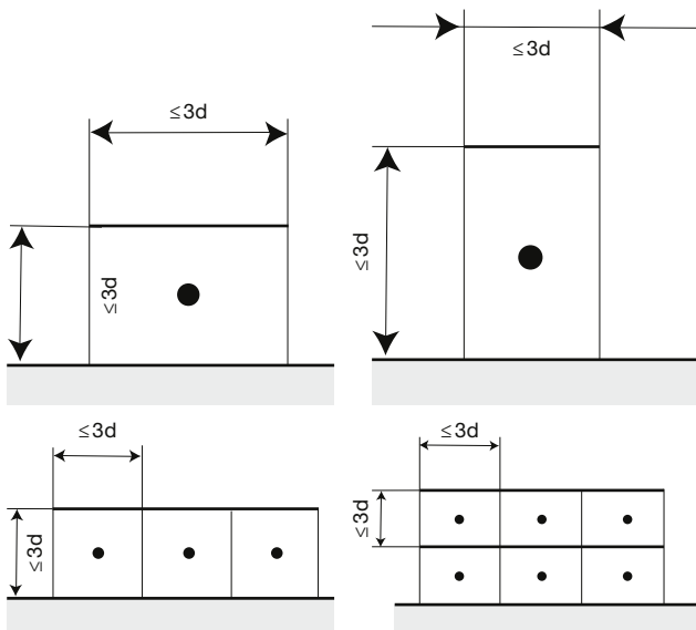
Fig.8 Définition des positions des microphones. d =distance de mesure par rapport au parallélépipède de référence.
