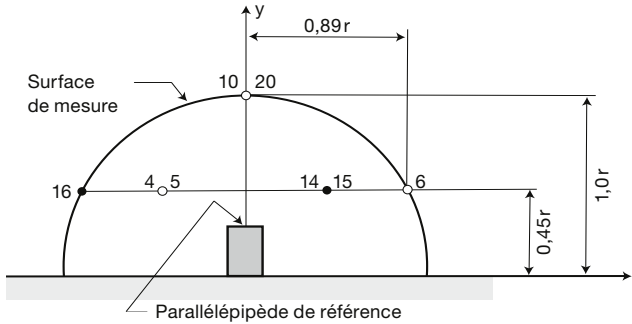
Fig. 7 Position de tous les microphones sur une surface de mesure hémisphérique (coordonnées: voir tableau 5). Ici, les points 14 à 16 et 20 sont des points de mesure supplémentaires.
