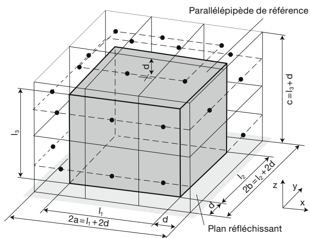
Fig. 13 Exemple de surface de mesure et de positions des microphones pour une grande machine.
