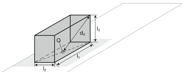
Fig. 3 Exemple pour un parallélépipède de référence sur un plan réfléchissant et distance caractéristique d_0 par rapport au centre du système de coordonnées.
