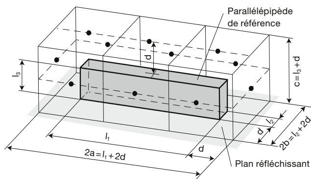
Fig. 11 Exemple de surface de mesure et de positions des microphones pour une machine longue.
