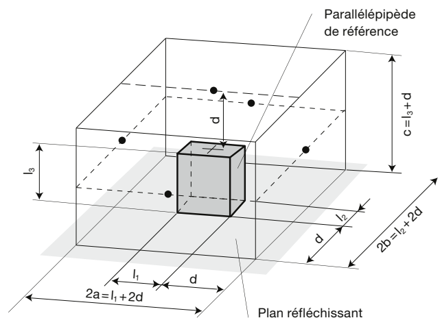
Fig.9 Exemple de surface de mesure et de positions des microphones pour une petite source de bruit.
