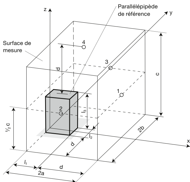
Fig. 14 Surface de mesure parallélépipédique avec quatre positions de microphones pour une source de bruit au sol et devant un mur [ S = 2(2ac + 2ab + bc) ].
