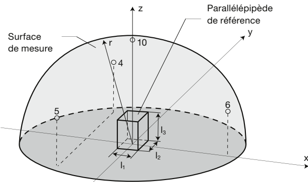
Fig. 6 Positions des microphones principaux 4, 5, 6 et 10 sur une surface de mesure hémisphérique (coordonnées: voir tableau 6).
