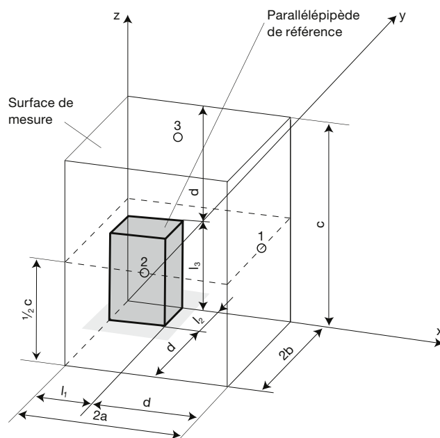
Fig. 15 Surface de mesure parallélépipédique avec trois positions de microphones pour une source de bruit au sol et devant un coin [ S = 2(ac + 2ab + bc) ].
