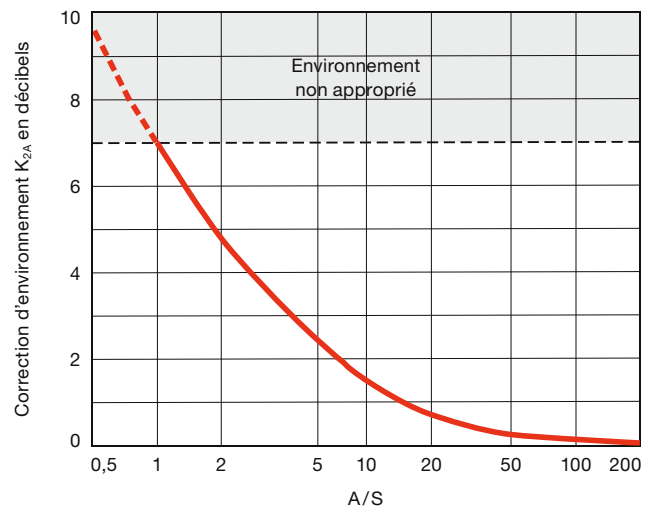
Fig. 17 Diagramme de correction d'environnement.
