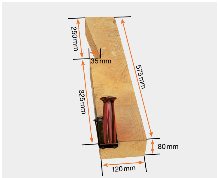
Fig. 16: dimensione dello spingitoio speciale per il taglio di cunei
