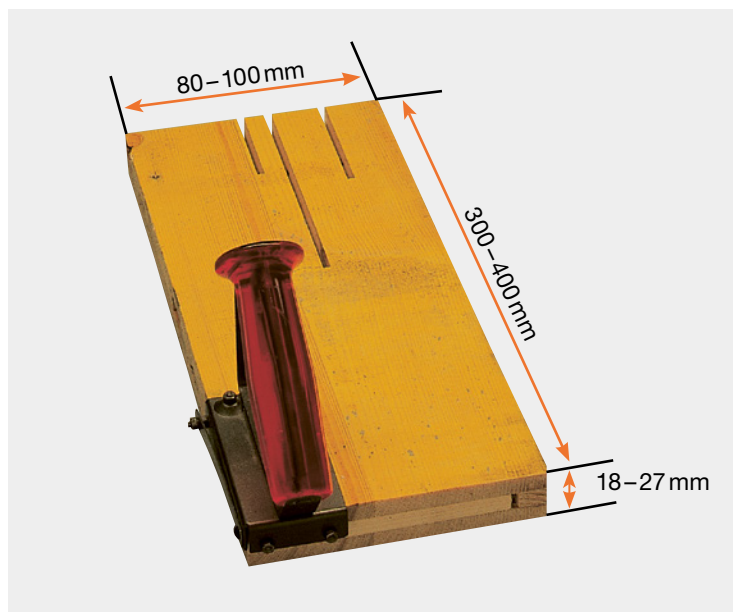
Fig. 11: dimensione dello spingitoio longitudinale
