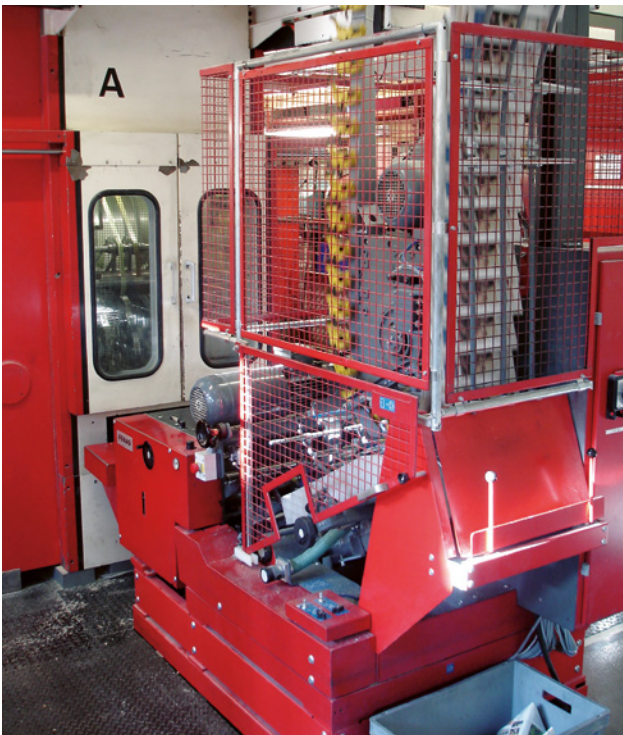
73 Impianto di imballaggio completamente incapsulato. La capsula riduce le emissioni sonore da 98 a 84 dB(A).
