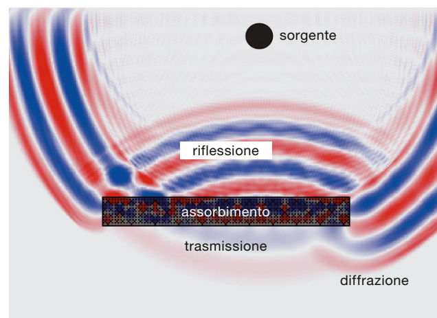
8 Risposte del suono a un ostacolo (grafico tracciato con il programma «Virtual Wave Tank»; Fraunhofer Institut für Integrierte Schaltungen, Dresda)
