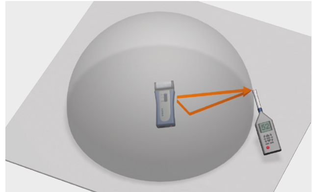
15 Sorgente sonora su una superficie piana, emissione semisferica
