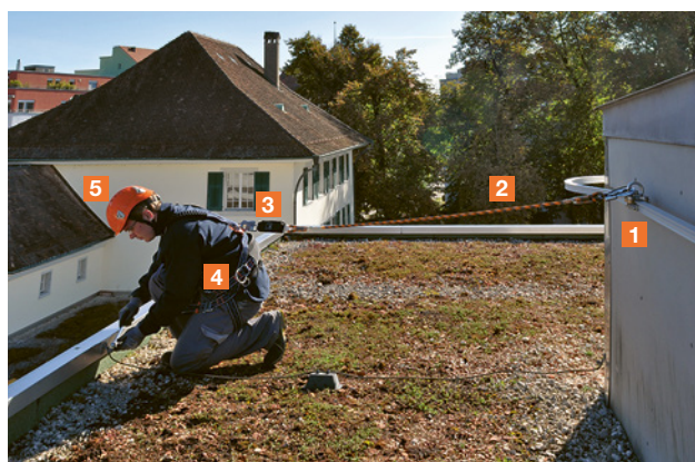
11 Rückhaltesystem auf einem Flachdach
