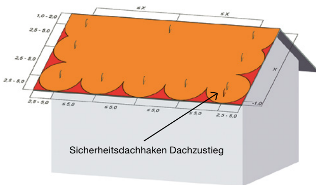
25 Satteldach mit Sicherheitsdachhaken
