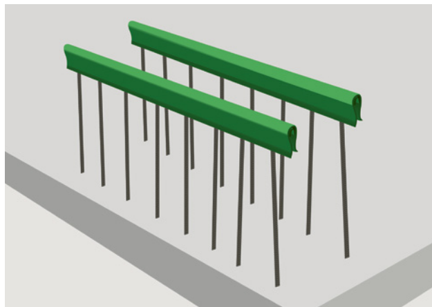
3 Rivestimento dei ferri di ripresa con profilo di sicurezza testato
