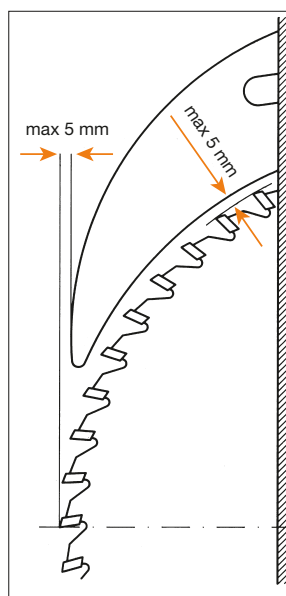
2 Coltello divisore in posizione di lavoro, allineato in modo corretto.
