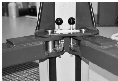
5 Dispositivo di sicurezza contro la rotazione dei bracci portanti.
