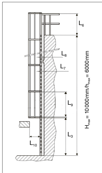
4 Vista laterale di una scala di accesso ai macchinari (figura: SN EN ISO 14122-4)
